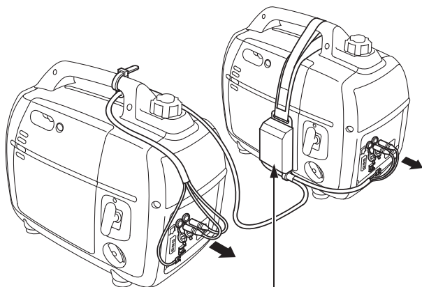
CAJA DE RECEPTÁCULOS PARA OPERACIÓN EN PARALELO (SE VENDE POR SEPARADO)
