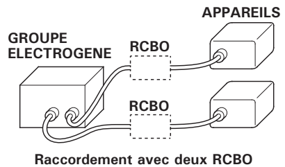
Raccordement avec deux RCBO
