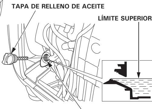
ORIFICIO DE RELLENO DE ACEITE
